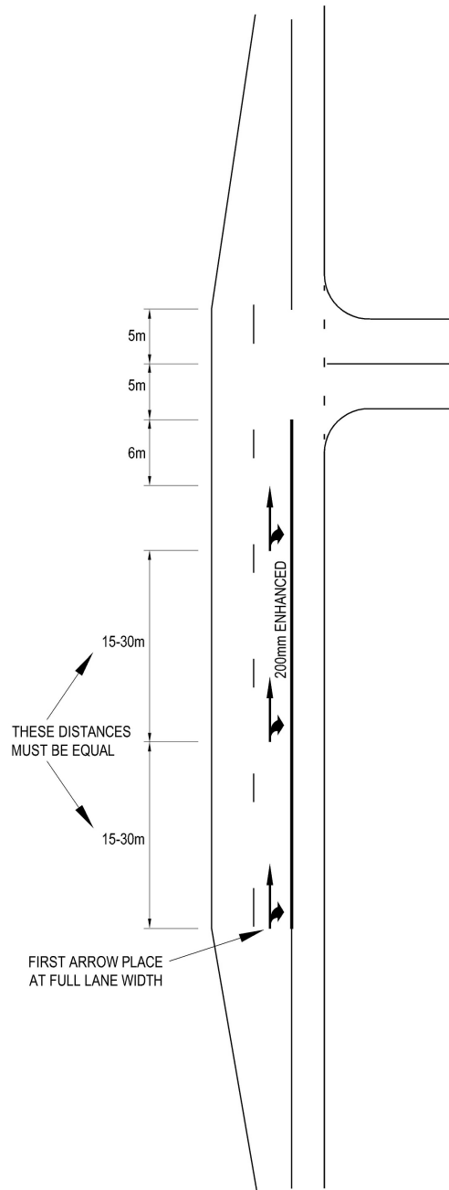
(d) BASic Right turn (BAR) For roads \leq 70 km/h
